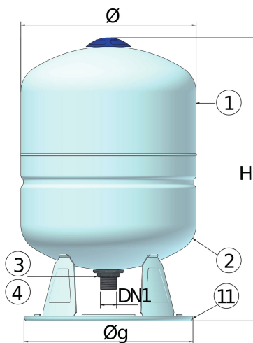
DPV 50 - 500
